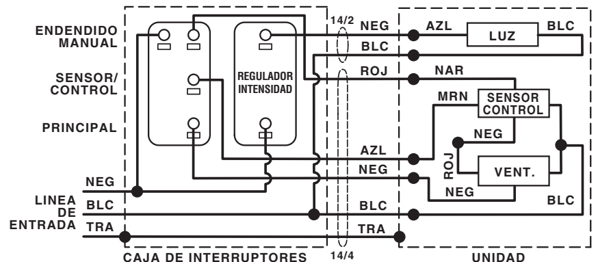
LUZ CON REGULADOR DE INTENSIDAD
